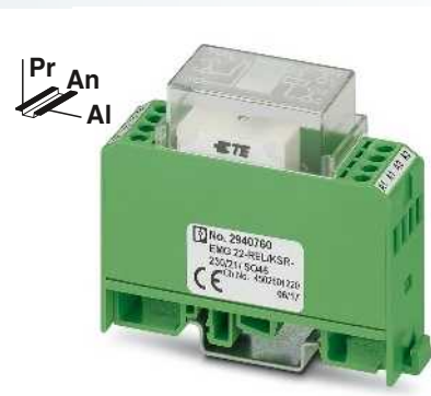
1 contacto conmutado, relé soldado
