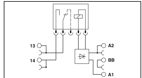
Módulo de relés de 1 contacto normalmente abierto con punto de embornaje libre de potencial adicional
