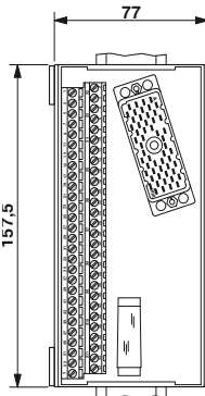
Esquema de dimensiones UMK-EC56/56-XOR
