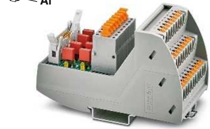
Módulo de fusibles para DeltaV para 8 canales con conexión push-in
