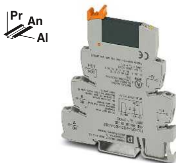
Módulo de relés de estado sólido, salida DC máx. 3 A
