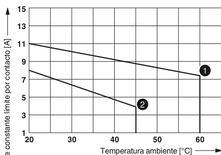
Contactos semejantes
