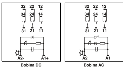
Módulo de relés de alta potencia de 3 contactos conmutados con conexión push-in
