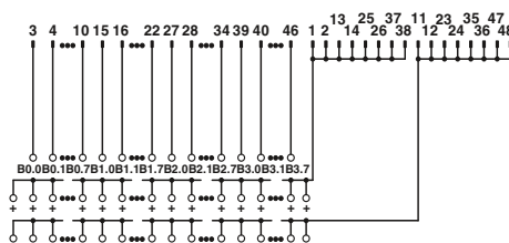
Esquema de conexiones FLKMS 50/32IM/PLC
