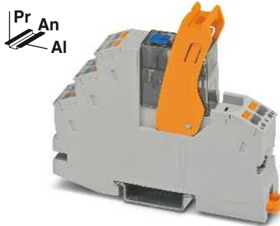
Módulo de relés de 2 contactos conmutados con conexión push-in y accionamiento manual
