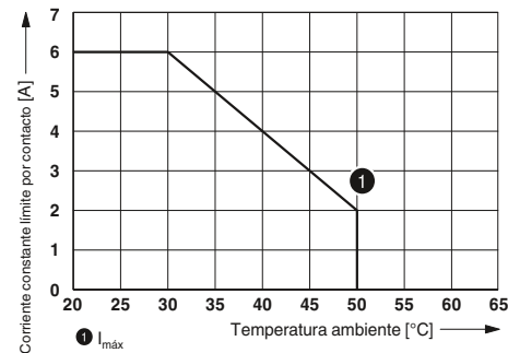
Contactos semejantes
