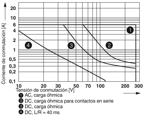
Capacidad de interrupción eléctrica para PLC...21HC/MS con 1 relé inversor
