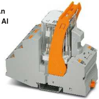
Módulo de relés de alta potencia de 2 contactos conmutados con conexión push-in
