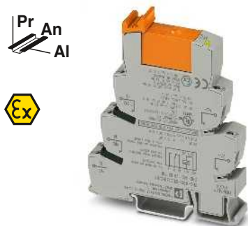
Módulo de relés de 1 contacto conmutado, máx. 10 A
