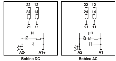
Módulo de relés de alta potencia de 2 contactos conmutados con conexión push-in
