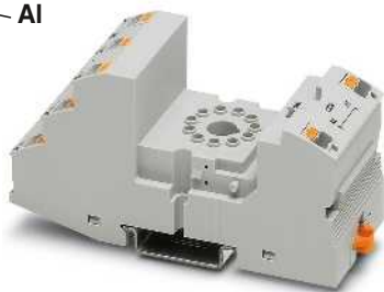
Zócalo de relé de 3 contactos conmutados con tecnología de conexión push-in para relés octales
