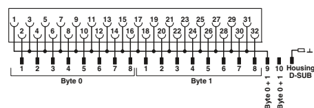
Esquema de conexiones FLKM-PA-2D15/HW/DI/C300
