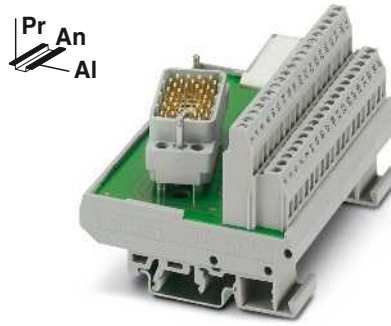
38 polos
