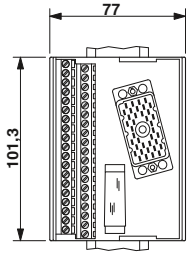
Esquema de dimensiones UMK-EC38/38-XOR
