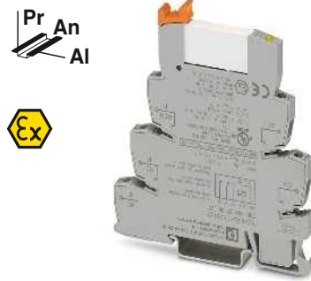
Módulo de relés de 1 contacto conmutado, máx. 6 A
