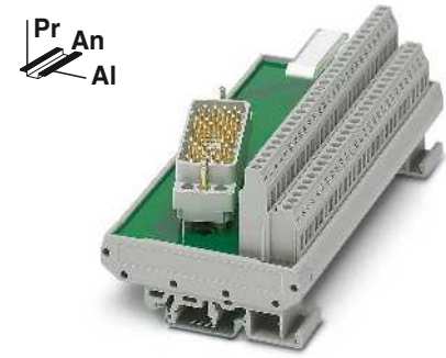
56 polos
