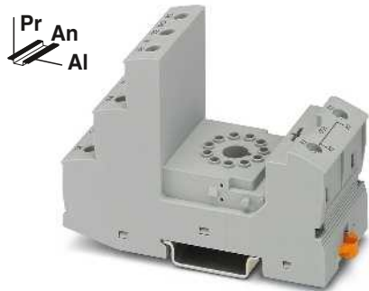
Zócalo de relé de 3 contactos conmutados con tecnología de conexión por tornillo para relés octales
