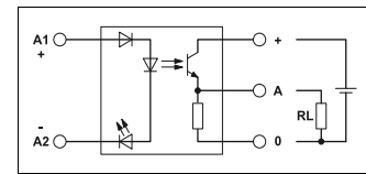
Figura 4: la salida de 3 conductores
