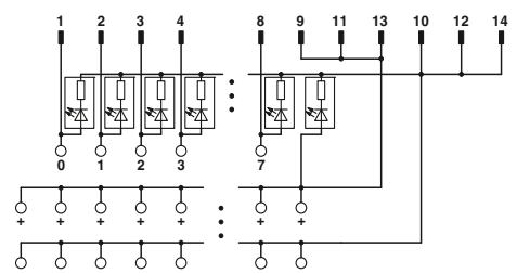
Esquema de conexiones VIP-3/.../FLK14/8IM/LED/PLC
