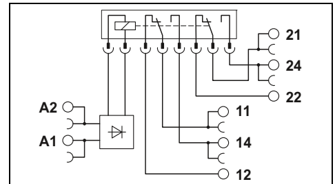
Módulo de relé de 2 conmutadores con accionamiento manual bloqueable, máx. 2 x 6 A
