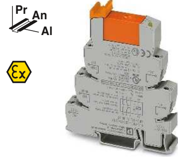
Módulo de relés de 2 contactos conmutados, máx. 2 x 6 A
