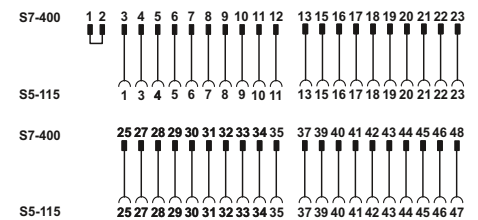
Esquema de conexiones FLKM S115/S400/SO155
