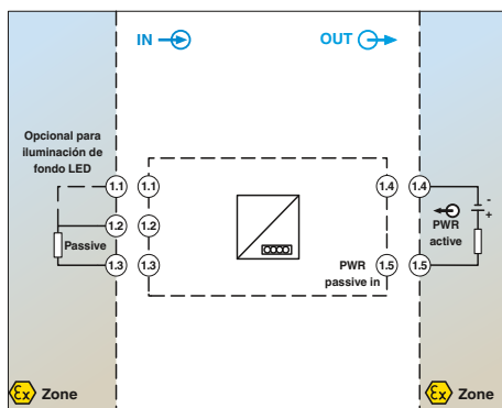
Esquema de conjunto FA MCR-EX-DS-I-I-OLP
