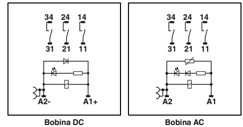
Módulo de relés de alta potencia de 3 contactos NA con conexión push-in
