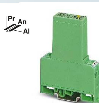
Relé de estado sólido de potencia máx. 2 A
