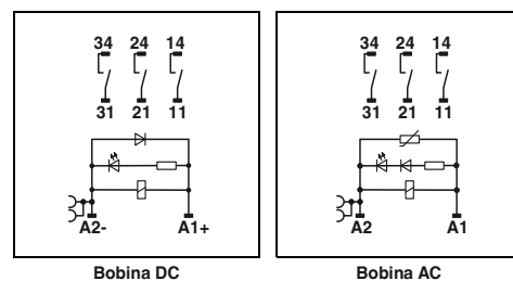
Bobina DC
