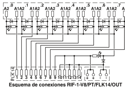
Esquema de conexiones RIF-1-V8/PT/FLK14/OUT
