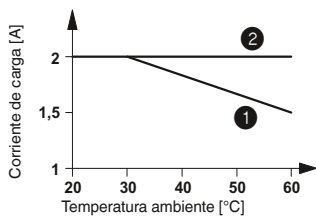
Curva derating para PLC-S...ELR W 1/2-24DC
