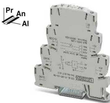
Relé temporizador con retardo de desco- nexión, con contacto de mando
