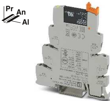
Módulo de relés de estado sólido con punto de embornaje libre de potencial adicional, salida DC máx. 100 mA
