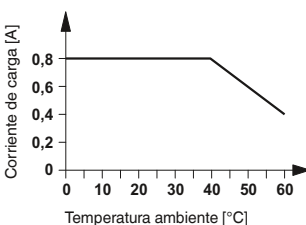
Curva derating para DEK-OV...240AC/800
