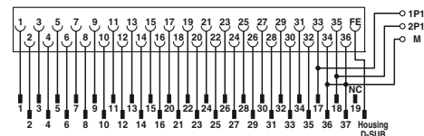
Esquema de conexiones FLKM-PA-D37/ETHA
