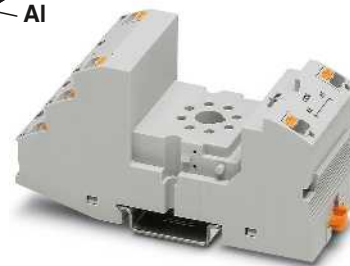
Zócalo de relé de 2 contactos conmutados con tecnología de conexión push-in para relés octales
