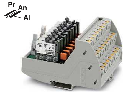
Módulo de salida con 8 relés miniatura, 1 contacto conmutado y fusible por circuito de salida
