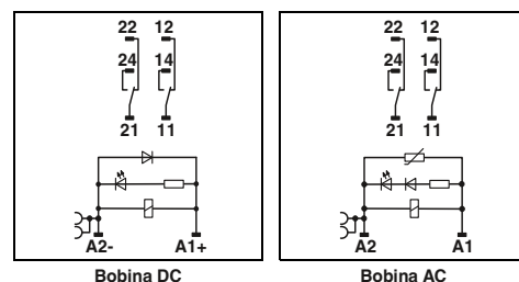
Módulo de relés de alta potencia de 2 contactos conmutados con conexión por tornillo
