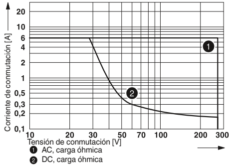
Capacidad de interrupción eléctrica para PLC...21 con 1 relé inversor
