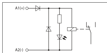
Construcción esquemática relé con entrada DC
