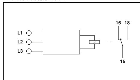
ERAC Ancho de la carcasa 17,5 mm
