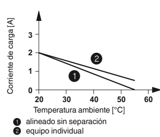
Curva derating para EMG 17-OV...48DC/2
