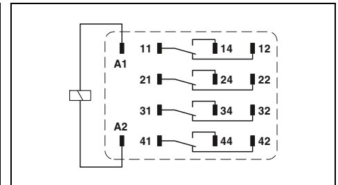
Relés industriales con cuatro conmutadores (sin polaridad) con accionamiento manual, máx. 4 x 6 A
