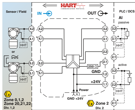
Amplificador separador de alimentación y entrada
