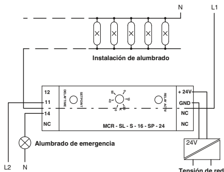
Instalación de alumbrado con alumbrado de emergencia
