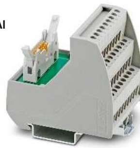
Módulo detector de 8 canales con conexión por tornillo
