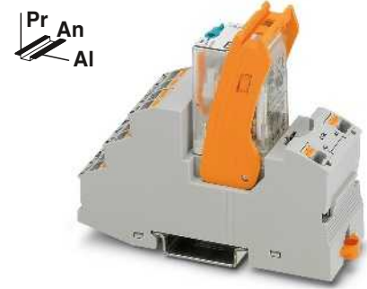
Módulo de relés industrial de 2 contactos conmutados con conexión push-in y accionamiento manual
