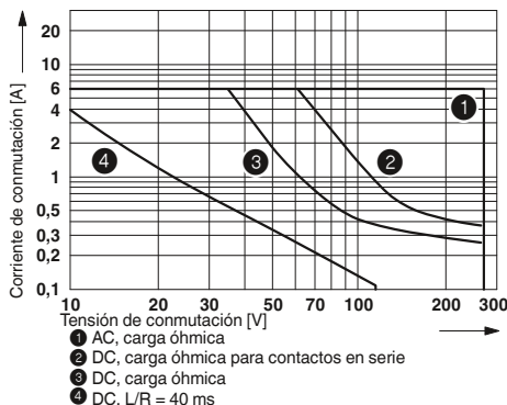
Potencia máxima de ruptura eléctrica para PLC...24DC/1-1/ACT con relés de 2 contactos normalmente abiertos
