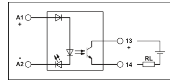
Figura 3: la salida de 2 conductores
